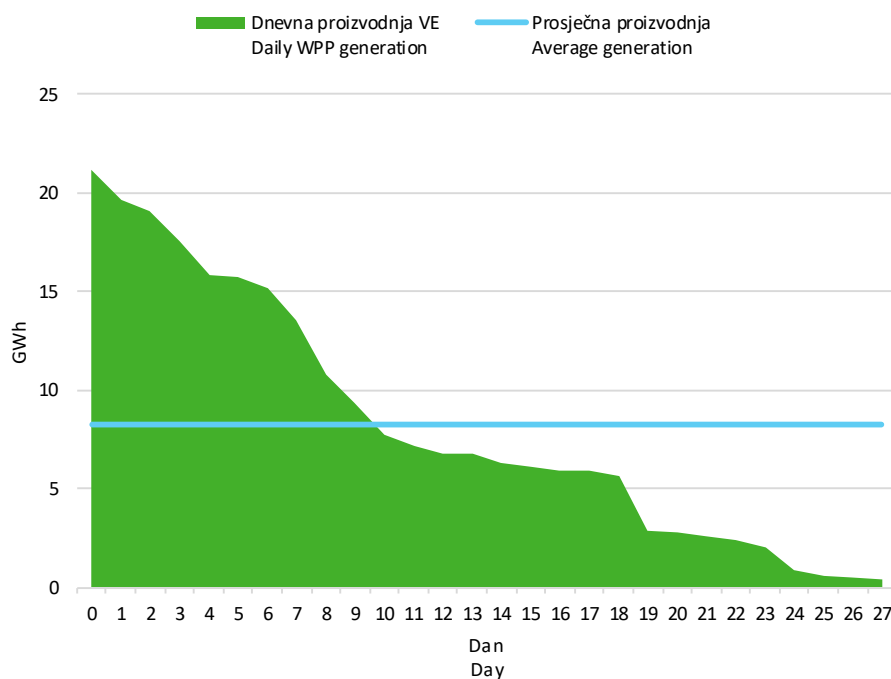
Slika 6 Krivulja trajanja dnevne proizvodnje vjetroelektrana u veljači 2026. godine
