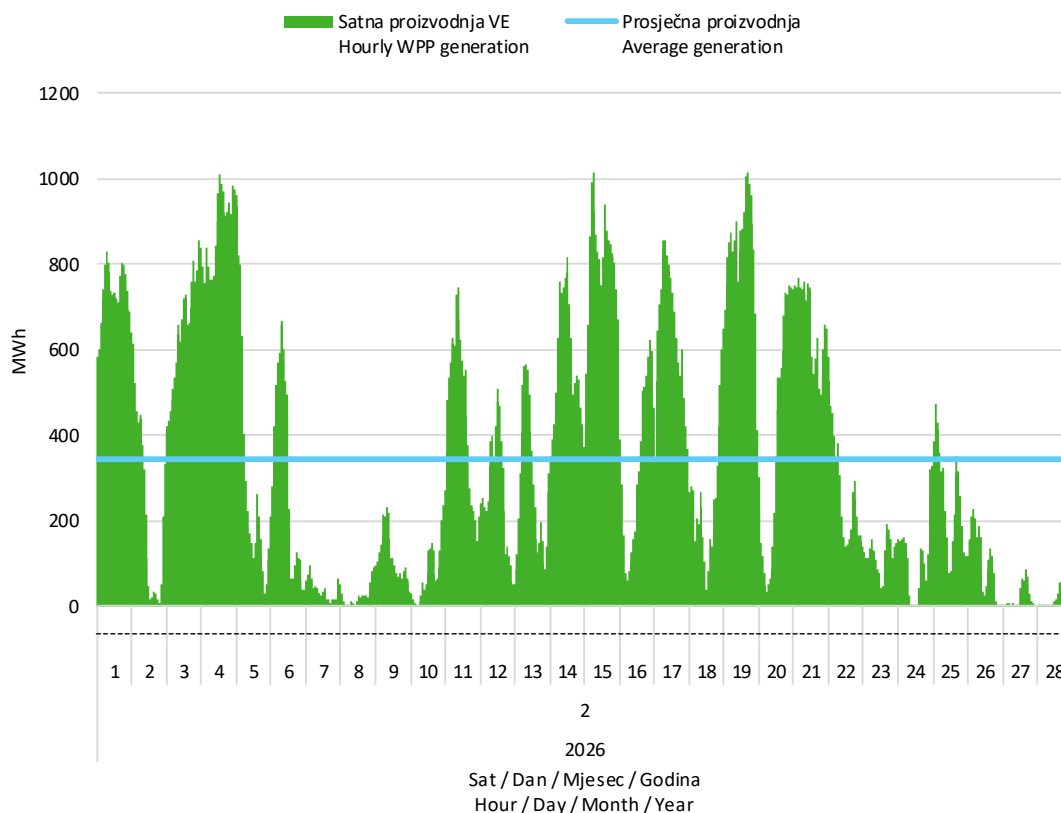
Slika 2 Satna proizvodnja svih vjetroelektrana u veljači 2026. godine
