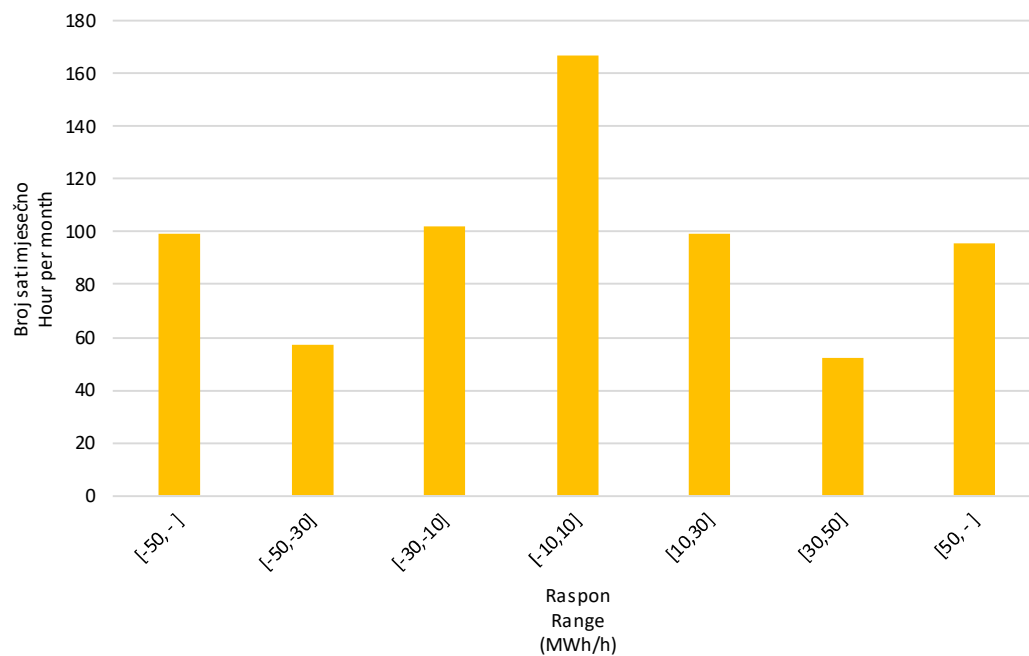
Slika 10 Statistička raspodjela satnih promjena proizvodnje VE u veljači 2026. godine
