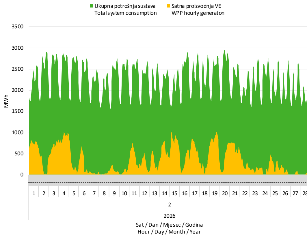
Slika 7 Usporedba satnog dijagrama opterećenja sustava i proizvodnje vjetroelektrana u veljači 2026. godine
