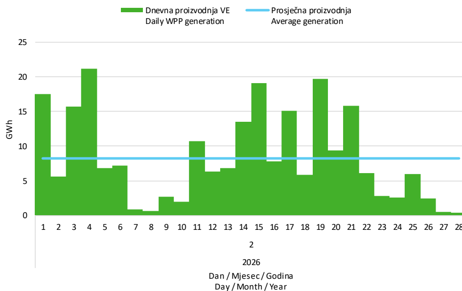
Slika 5 Dnevna proizvodnja svih vjetroelektrana u veljači 2026. godine
