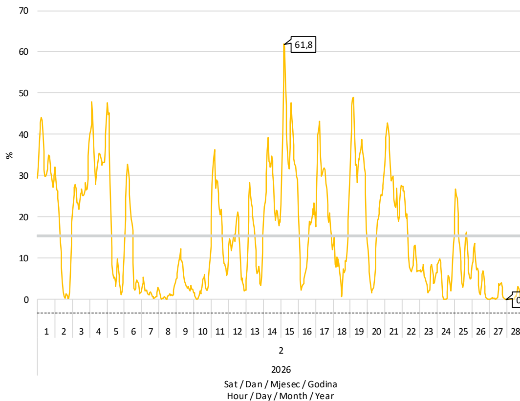
Slika 8 Udio proizvodnje vjetroelektrana u pokrivanju satnog opterećenja elektroenergetskog sustava u veljači 2026. godine
