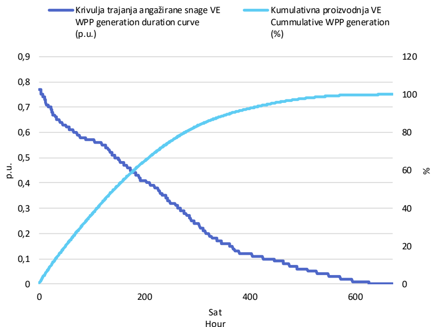
Slika 3 Krivulja trajanja angažirane snage svih VE i kumulativna proizvodnja VE u veljači 2026. godine u jediničnim vrijednostima
